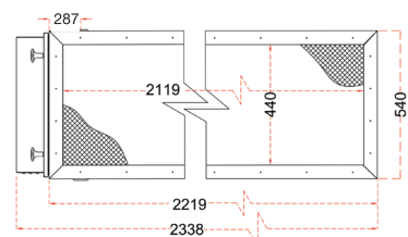
Mặt cắt cửa hút khí
