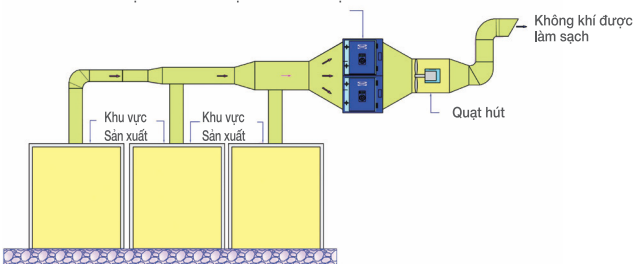
Thiết bị lọc không khí công nghệ tĩnh điện RY2500B hoặc RY5000B hoặc RY7500B hoặc RY10000B
